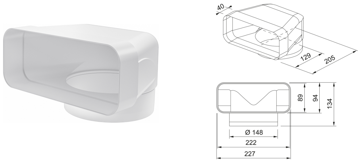
Pièce de dérivation F-UR 150 90°
