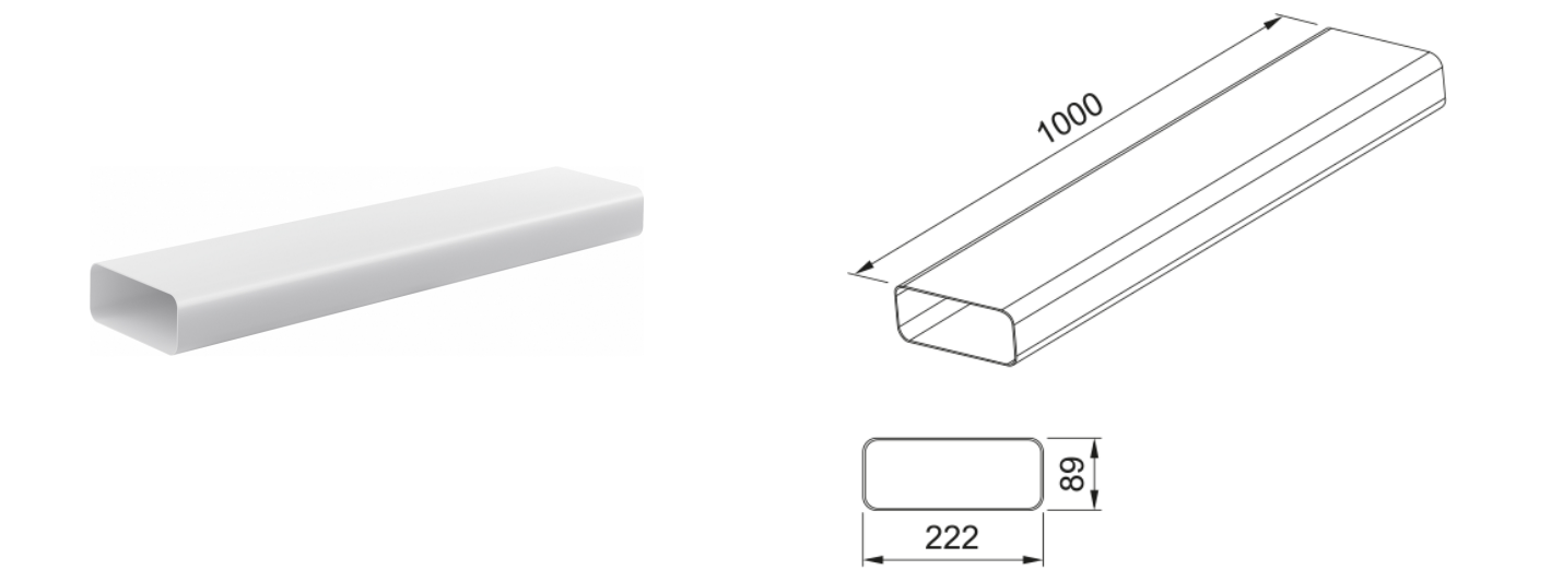
GAINE DE CONDUITE PLATE F-VRO 150 POUR TABLES ASPIRANTES
