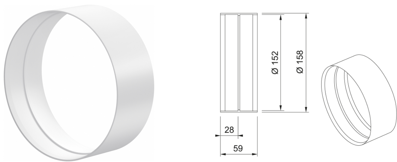
Connecteur de tuyau R-VBS 150 im 155 mm Long 60 mm
