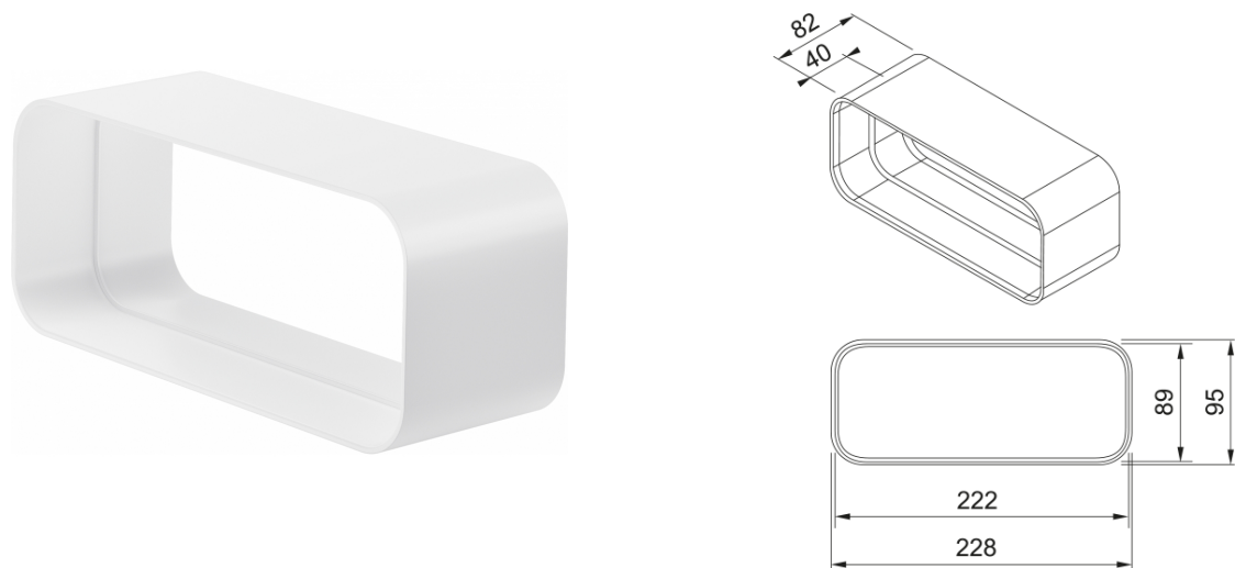
Connecteur de tuyau F-RVB 150 Forme angulaire
