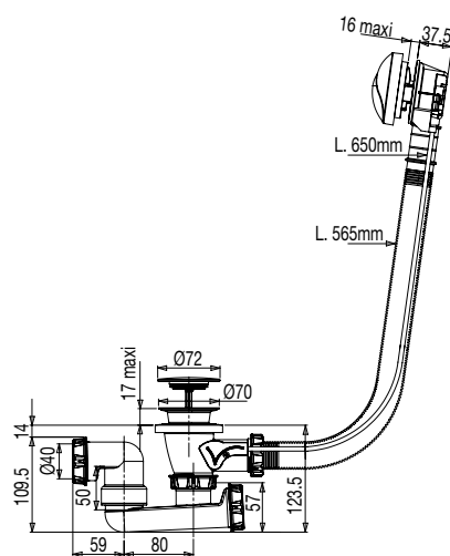
Volant et grille de trop-plein autocentable
