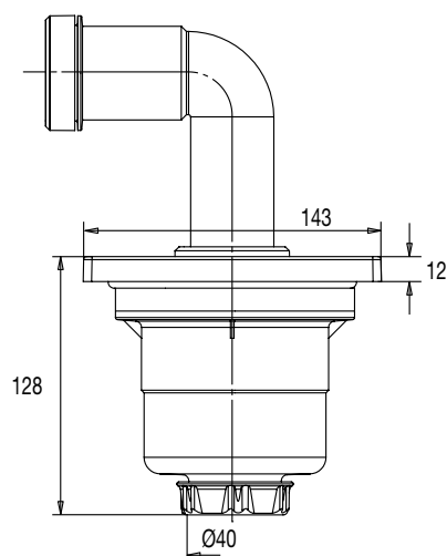
Aménagement douche de plain- pied
