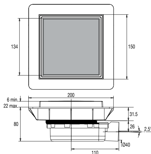
Cadre à carreler ajustable
