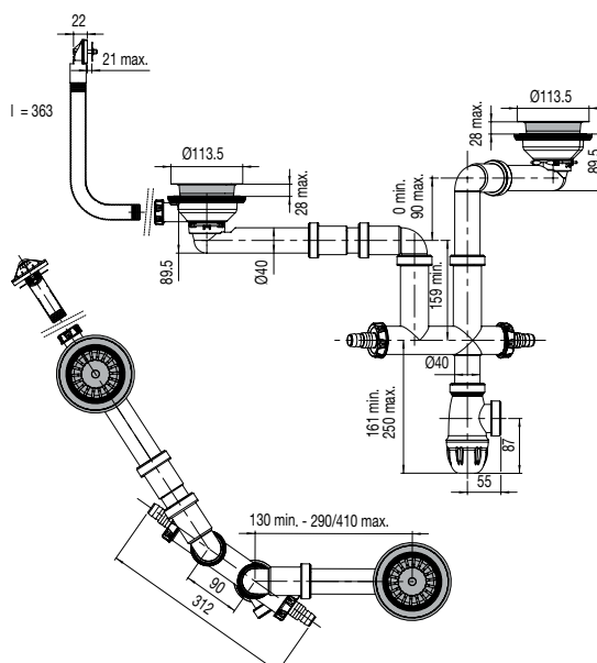
Joint autofix maintenu sur bonde
