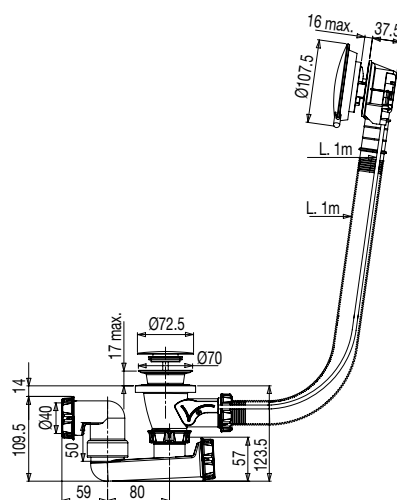
Volant et grille de trop-plein autocentrable
