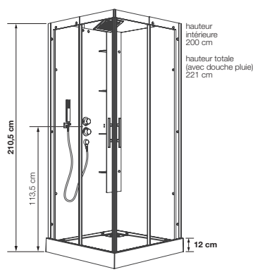
Cotes pour le modèle C80
