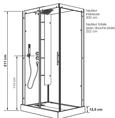
Cotes pour les modèles 110x81, 120x91 et C90
